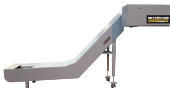
Dopravníky triesok
